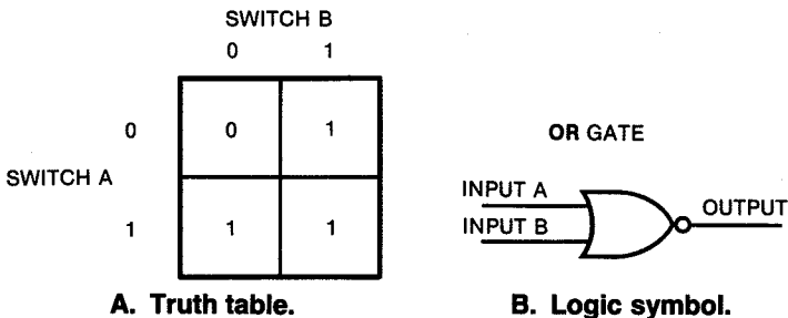
Fig. 1-8. An OR gate.
